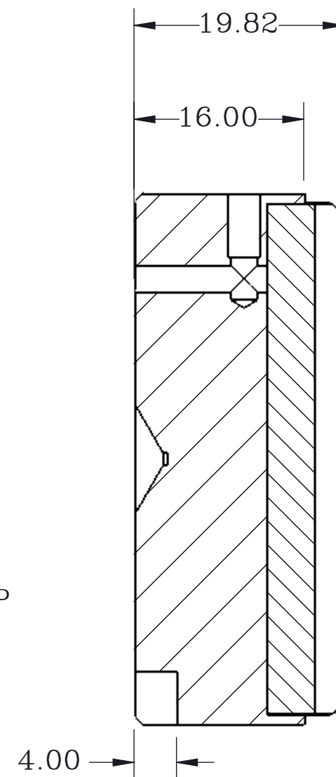
SECTION A-A
