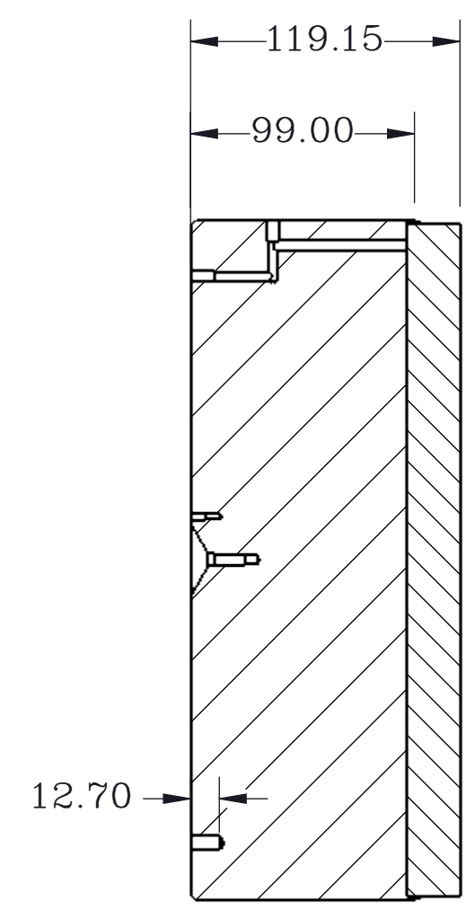
SECTION A-A
